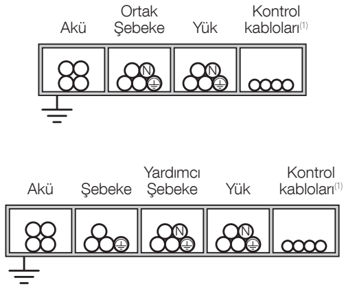
Doğru montaj
